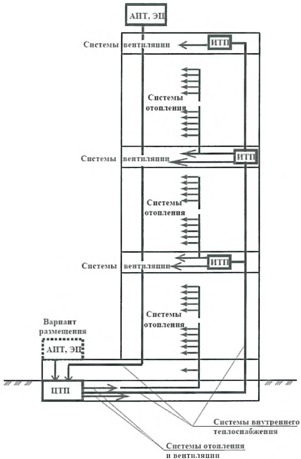
Рисунок 5.2 – Схема теплоснабжения высотного здания от автономного источника (АНТ, ЭЦ)
